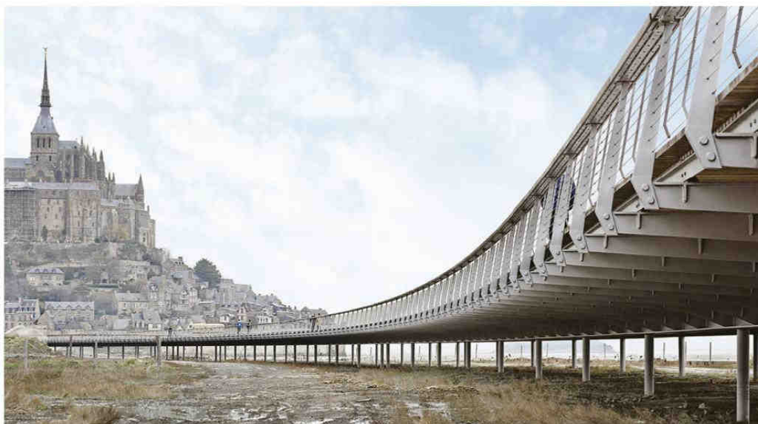
Ouvrages d'art « La Jetée », accès au Mont-Saint-Michel (Manche) Maitre d'ouvrage: Syndicat mixte Baie du Mont-Saint-Michel Concepteurs: Dietmar Feichtinger Architectes avec Schlaich Bergermann und Partner
